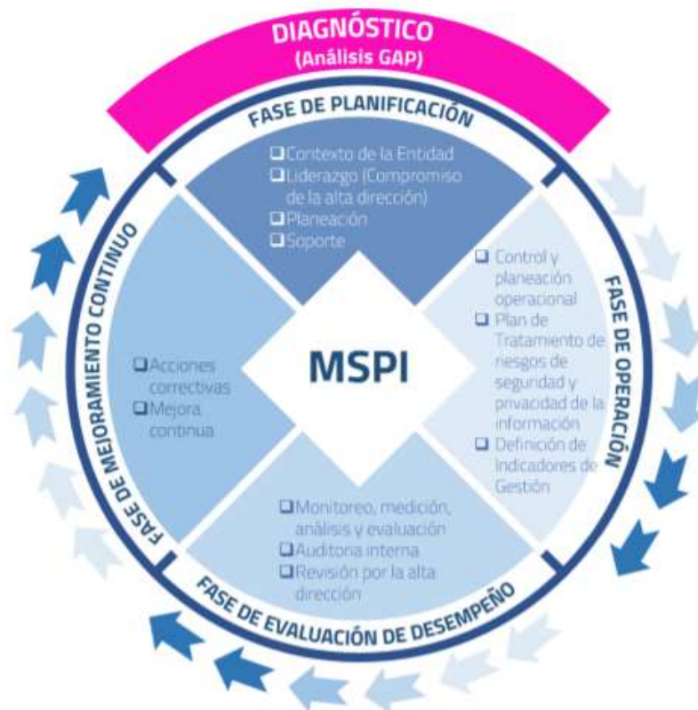
Ilustración 1 - Metodología MSPI
